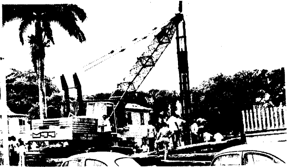
De machine van N.V. Exploitatie Mij bezig met het heien van de eerste paal. Dokter Jamaludin verlaat de cabine.
